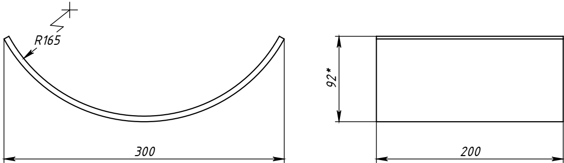
Поз.3 (Ложемент)
